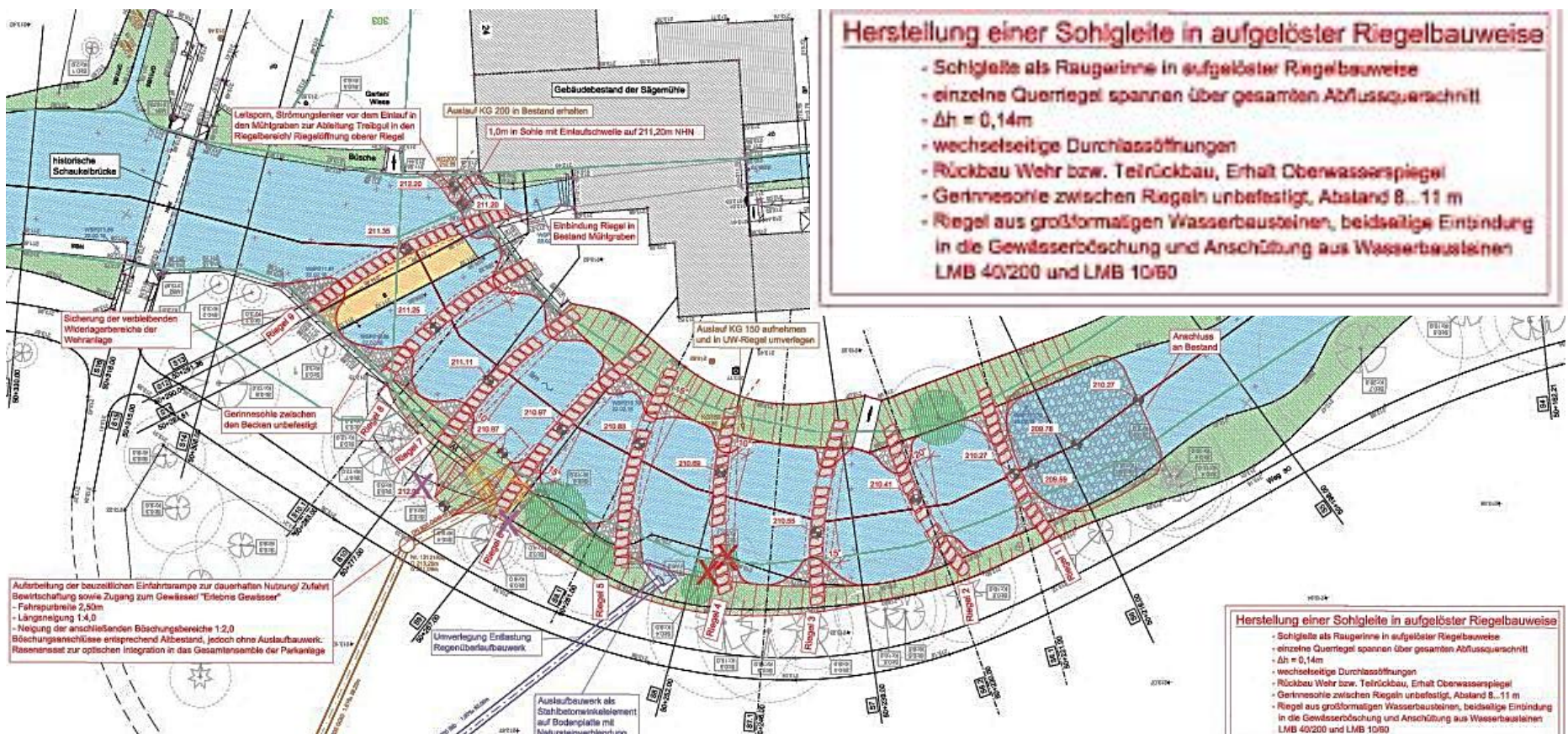
Abb. 1: Lageplan Zielzustand/ Vorzugsvariante: Sohlgleite in aufgelöster Riegelbauweise zur ökologischen Durchgängigkeit des Wehr an der Sägemühle
